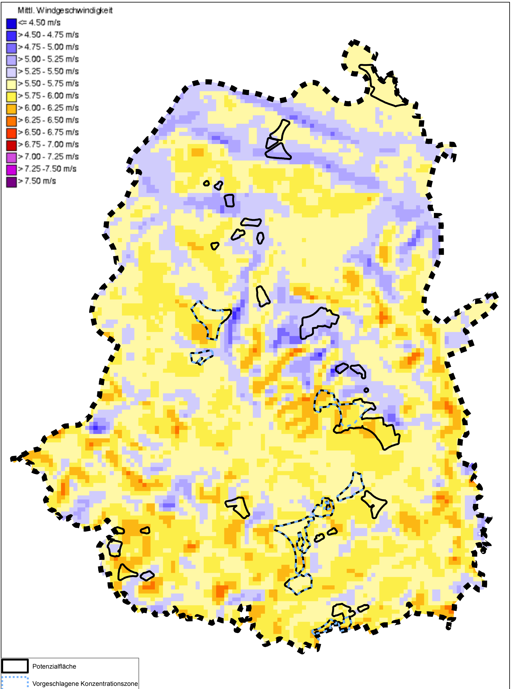
Karte 5 Windgeschwindigkeiten in 100 m über Grund
