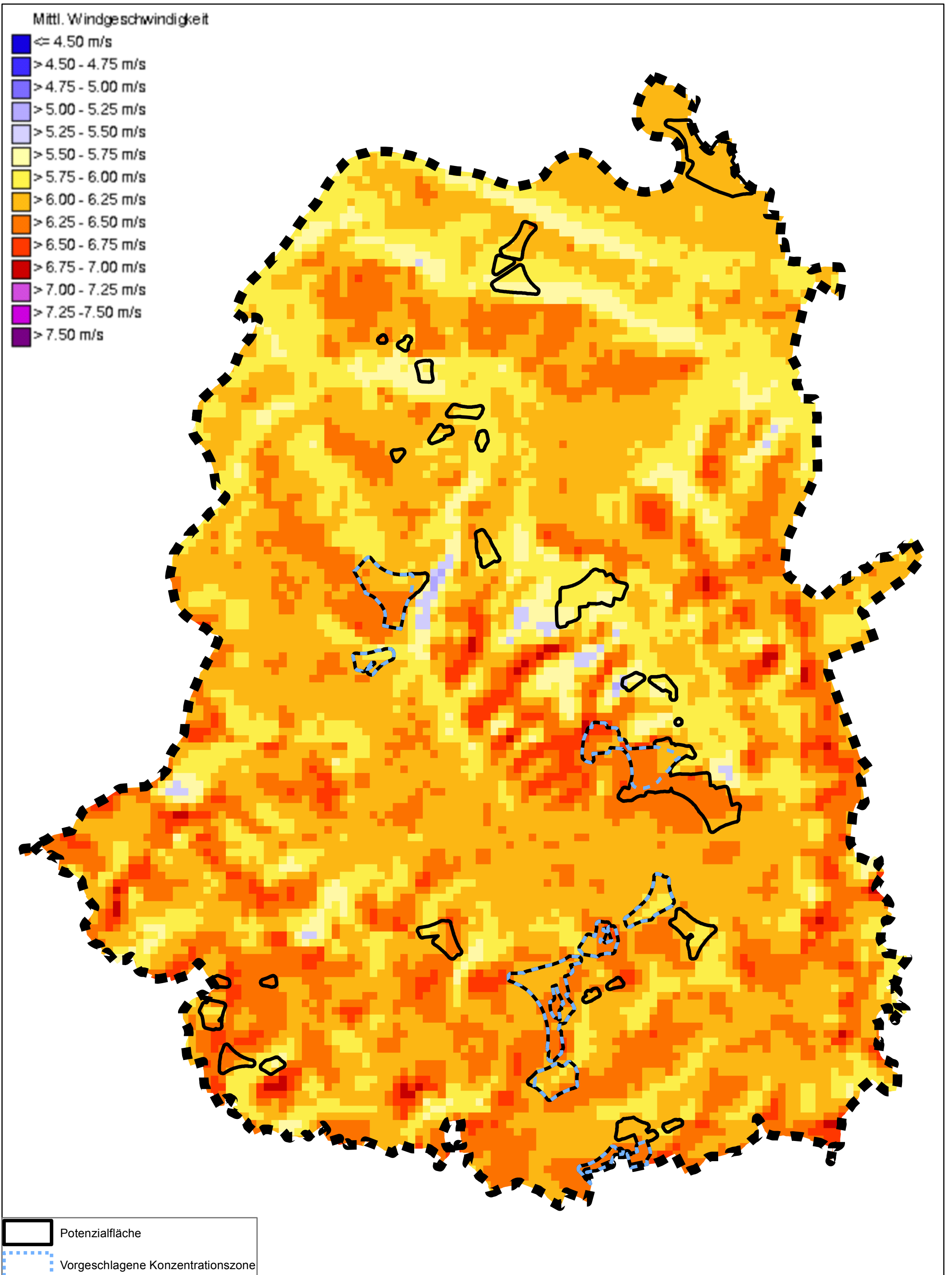
Karte 6 Windgeschwindigkeiten in 125 m über Grund
