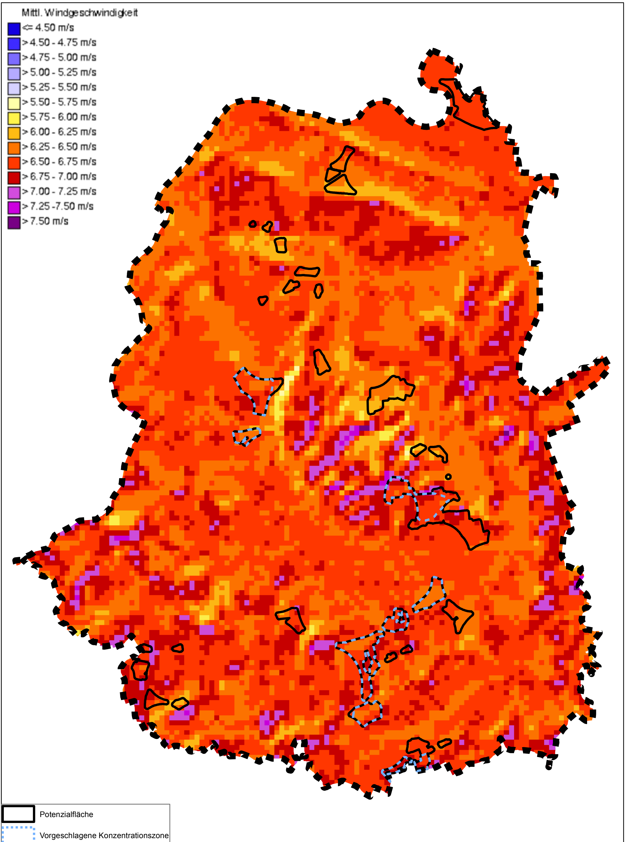
Karte 8 Windgeschwindigkeiten in 150 m über Grund
